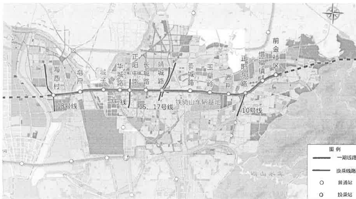
图 1 青州市地铁 9 号线一期工程线路示意图
